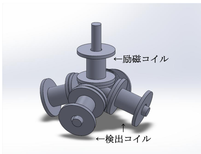
図 6 3D CAD で製作したボビン
