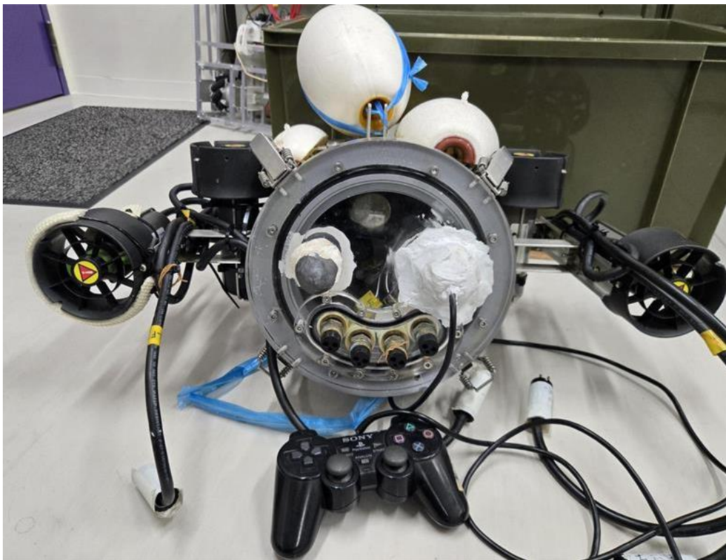
図 5 水中ドローン
